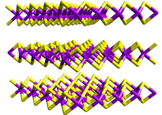
Chalcogenides
